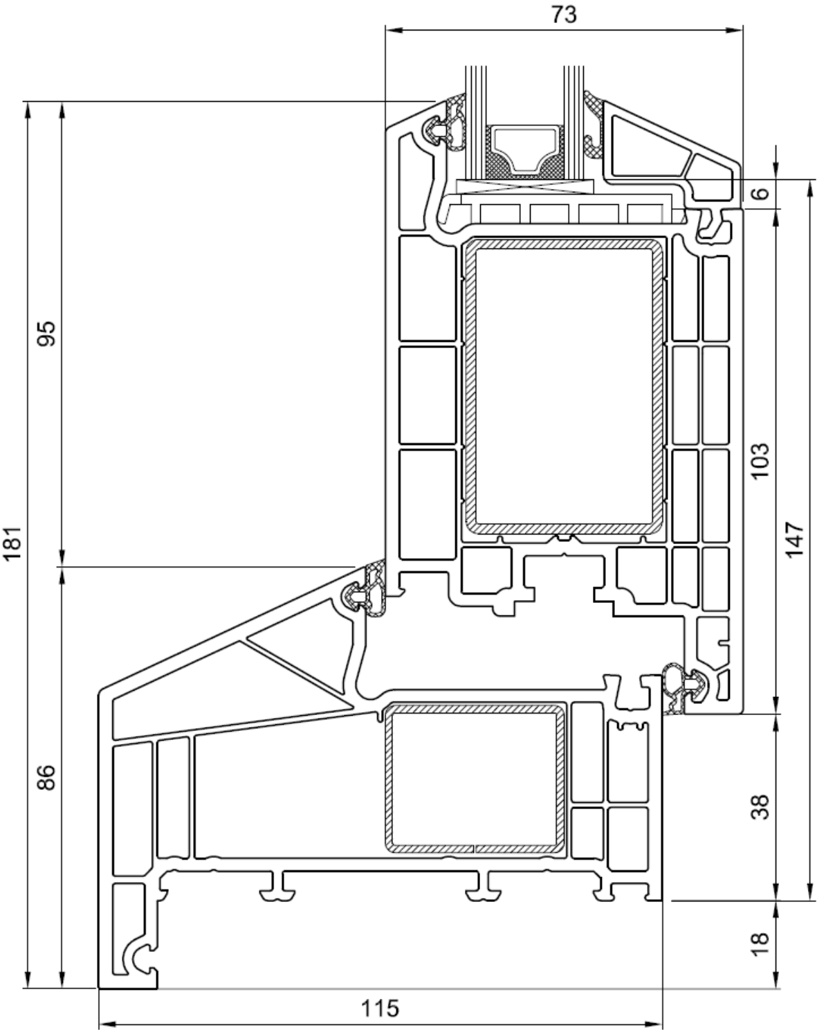
Kozijn met aanslag en deur binnen draaiend "verdiept profiel Creon"
