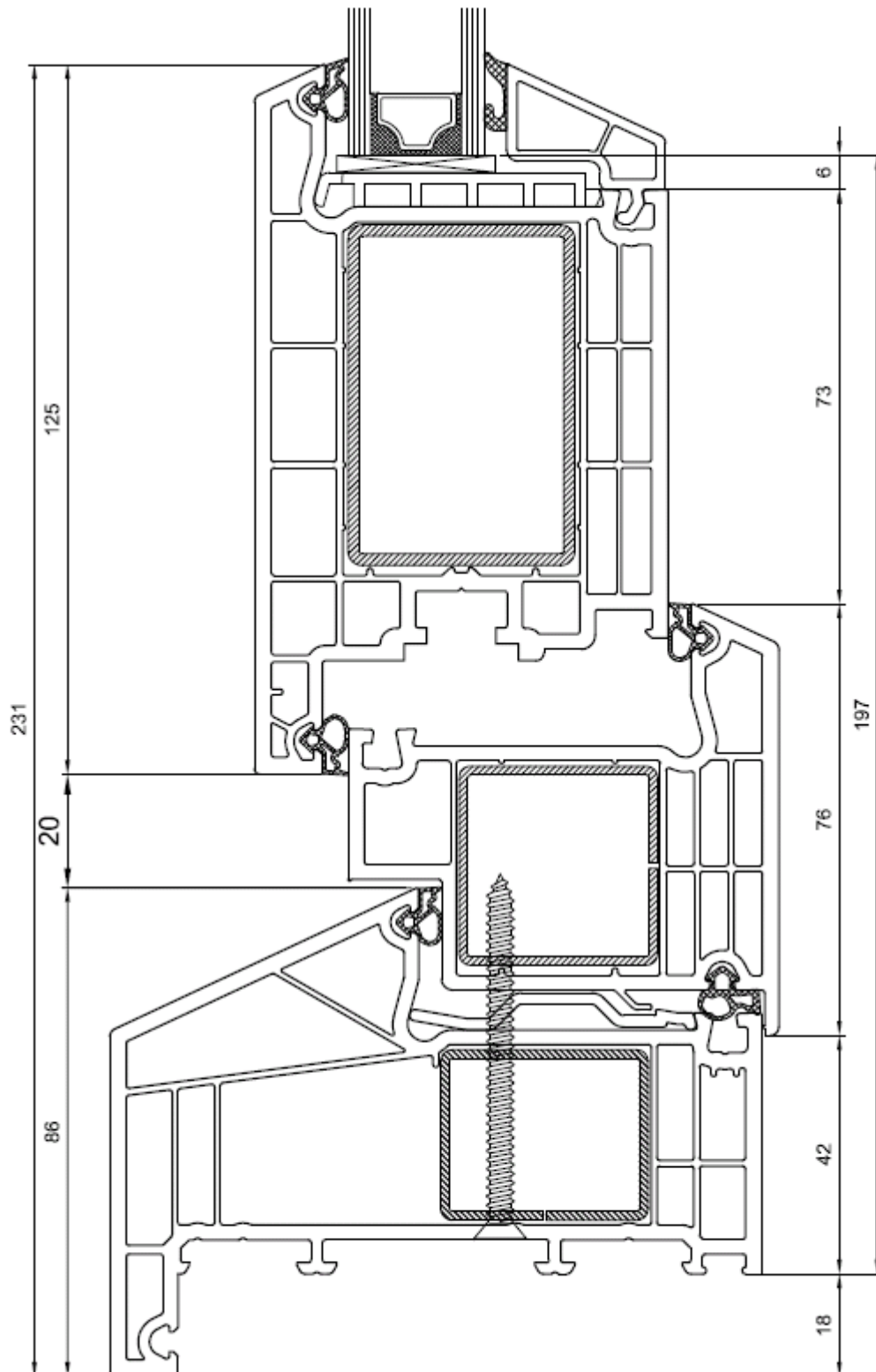
Kozijn met aanslag en deur buiten draaiend "verdiept profiel Creon"
